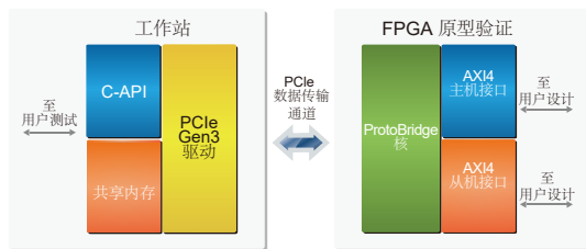
ProtoBridge AXI 架构
